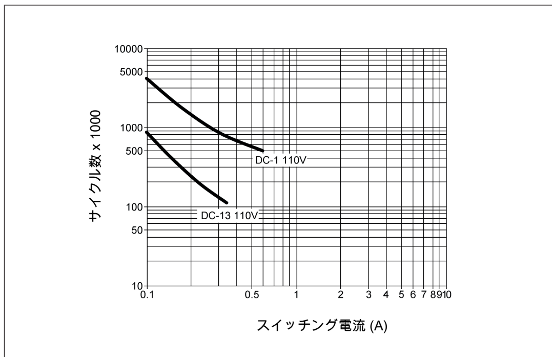
図: 製品寿命グラフ (110 V DC)
