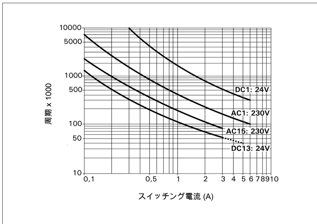
図: 製品寿命グラフ (24 V DCおよび230 V AC)
