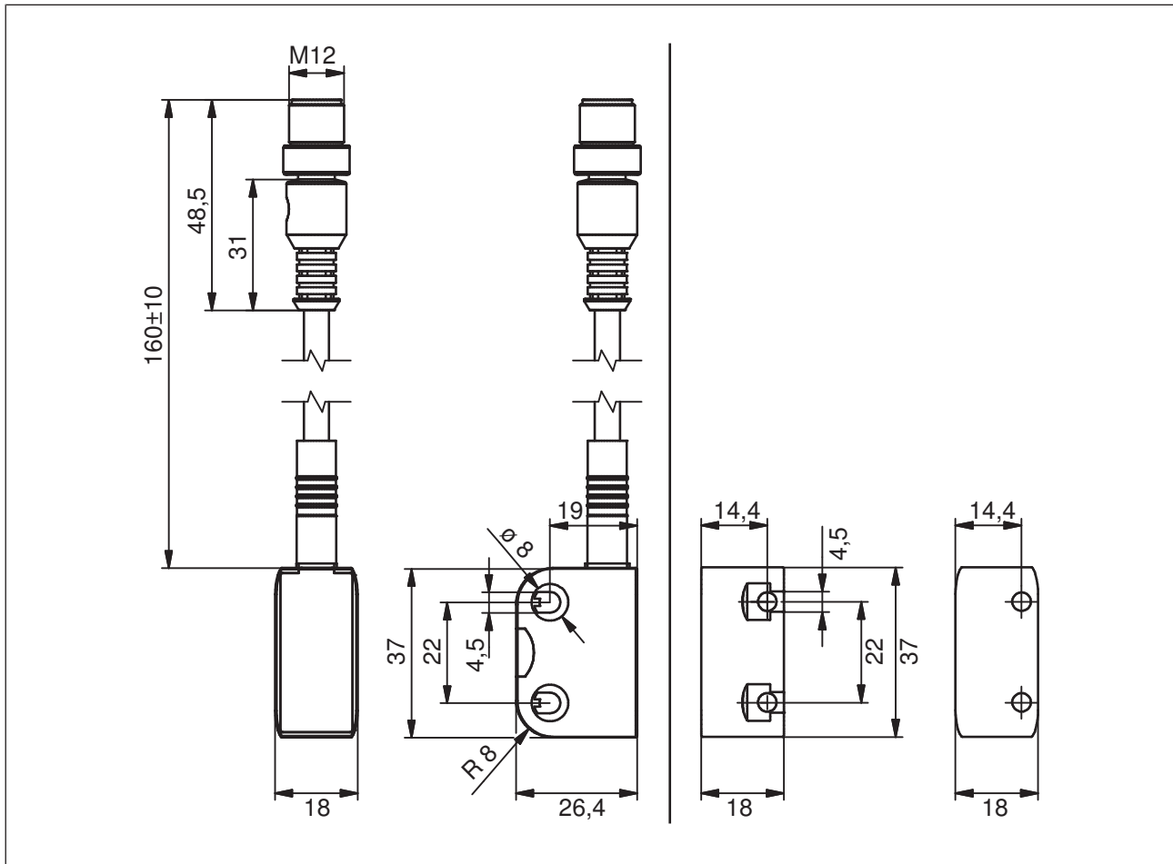
図: 安全スイッチ (左) およびアクチュエータ (右)
