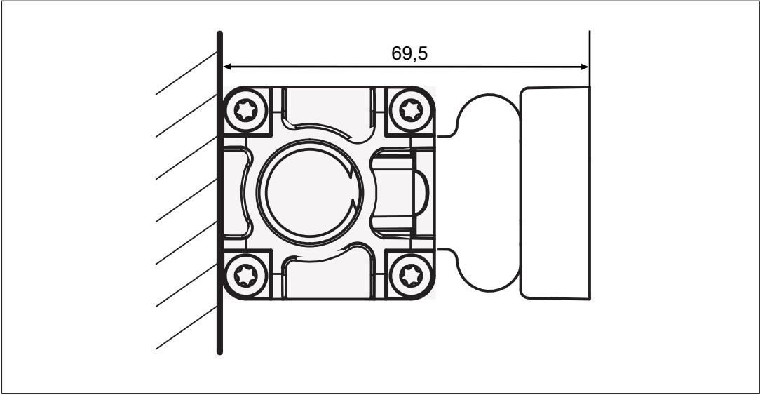
安全スイッチの取り付け面とアクチュエータの取り付け面の間の距離
